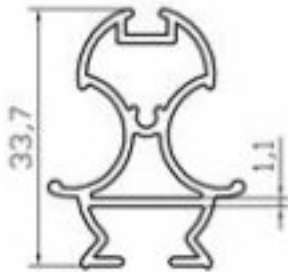
K4402 FİTİLLİ DİKME (KAYAR) (0.420 Kg/m)
