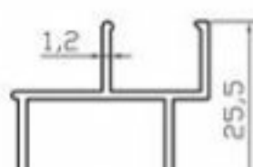
K4414 KAPI KARŞILIĞI (0.225 Kg/m)
