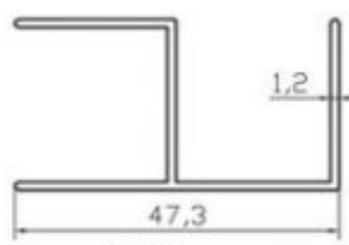
K4411 DİKME BAĞLANTI (0.395 Kg/m)
