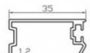
K4416 DIŞ RAY PROFİLİ (0.325 Kg/m)
