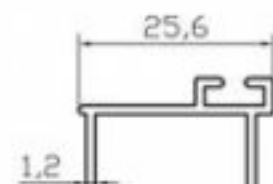
K4425 KAPI KARŞILIĞI (0.225 Kg/m)
