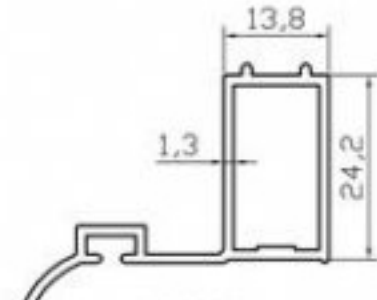
K4404 KAPI KARŞILIĞI (0.440 Kg/m)
